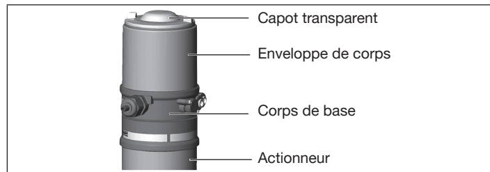
Fig. 34 : Ouvrir l'appareil
