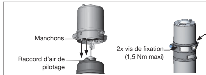
Fig. 11 : Montage
