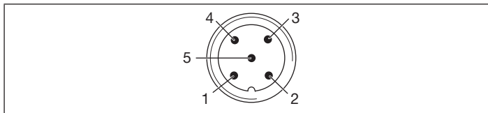
Fig. 22 : Affectation des raccordements
