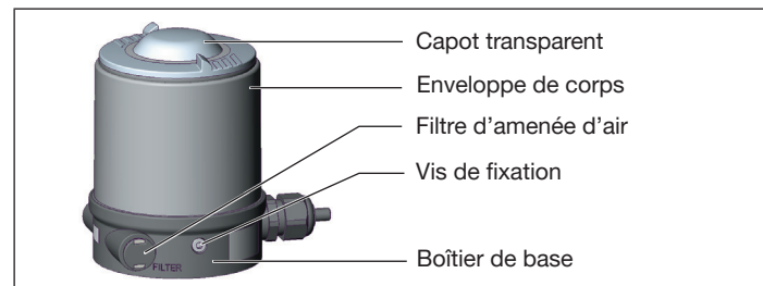
Fig. 2 : Construction, conduite d'air de pilotage intégrée
