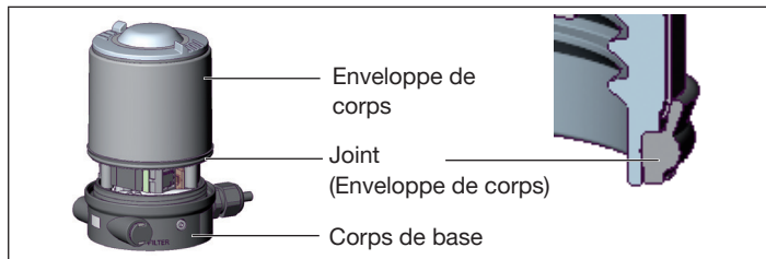
Fig. 37 : Fermer l'appareil
